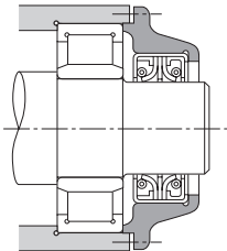
Рис.11.9. Пример применения масляного уплотнения (2)
