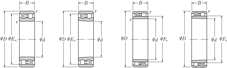
NN Цилиндрическое отверстие NN Коническое отверстие NNU Цилиндрическое отверстие NNU Коническое отверстие
