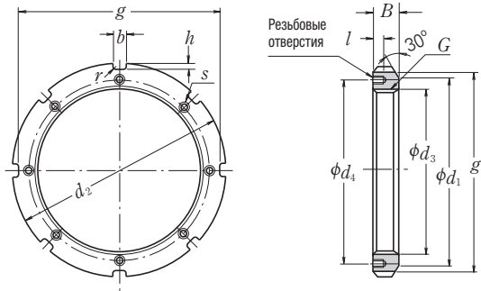
Гайка и фиксирующее устройство
