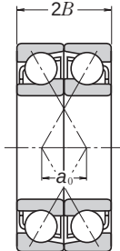
По X-образной схеме DF
