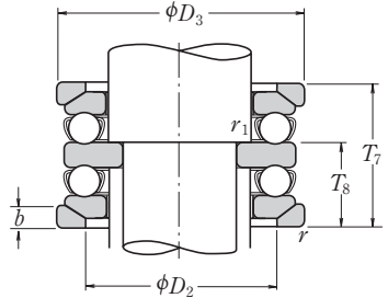
Со сферическим подкладным кольцом
